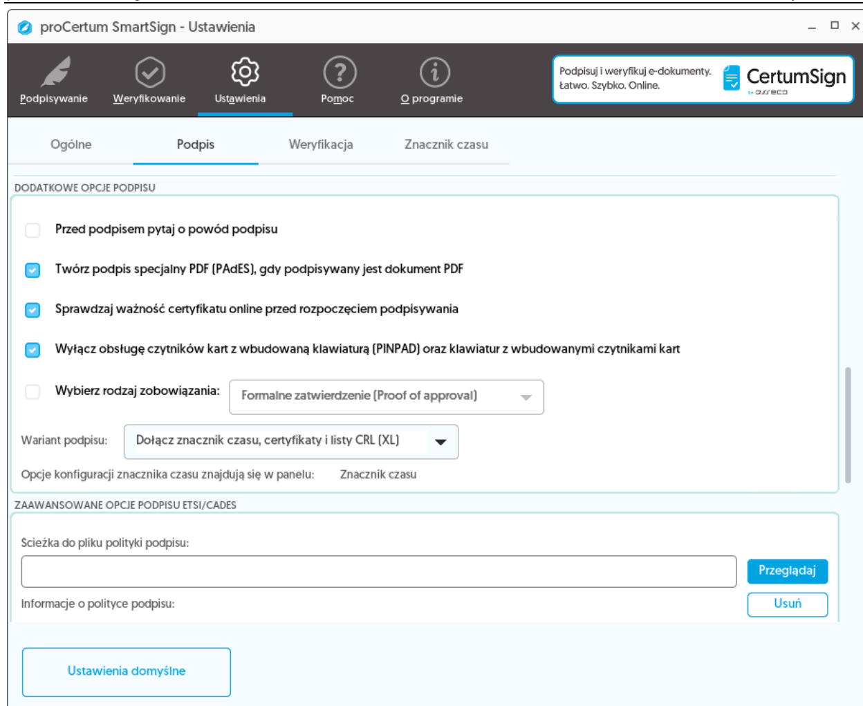
Rysunek 9: Zakładka Ustawienia – Podpis – część dotycząca zaawansowanych opcji podpisu
