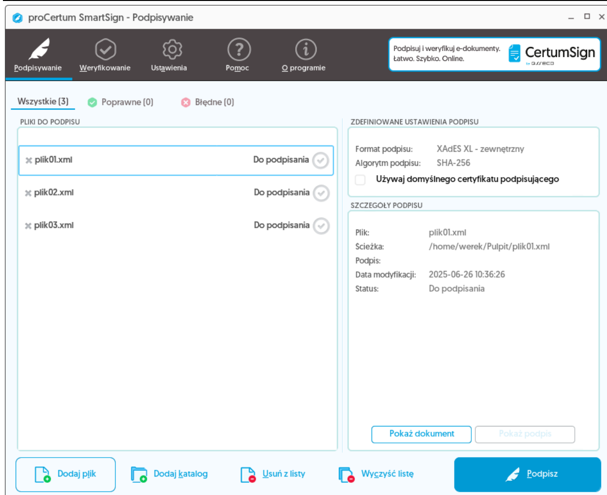
Rysunek 16: Zakładka Podpisywanie – Lista elementów do podpisania
