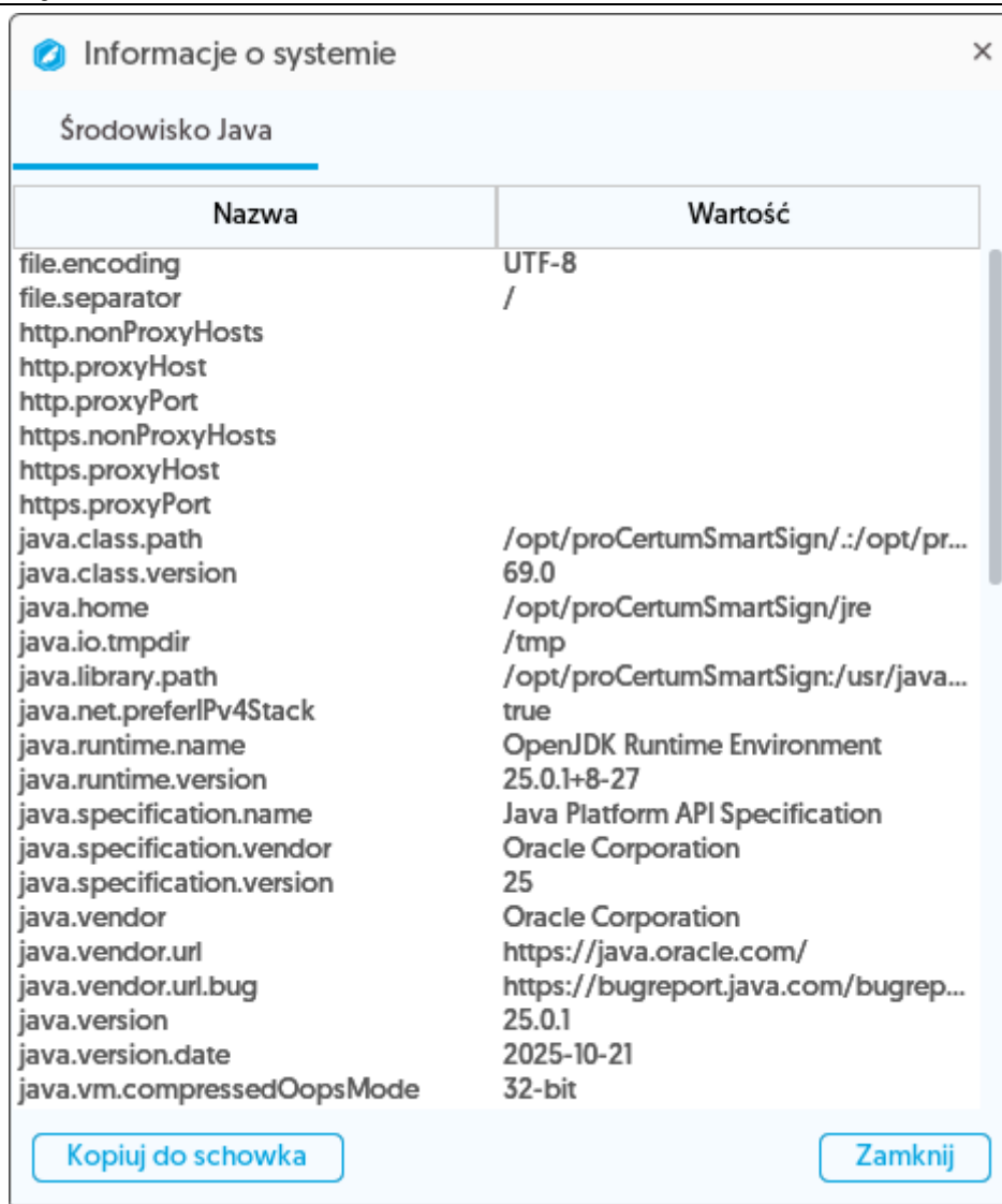
Rysunek 2: Informacje o systemie– Zakładka Środowisko Java
