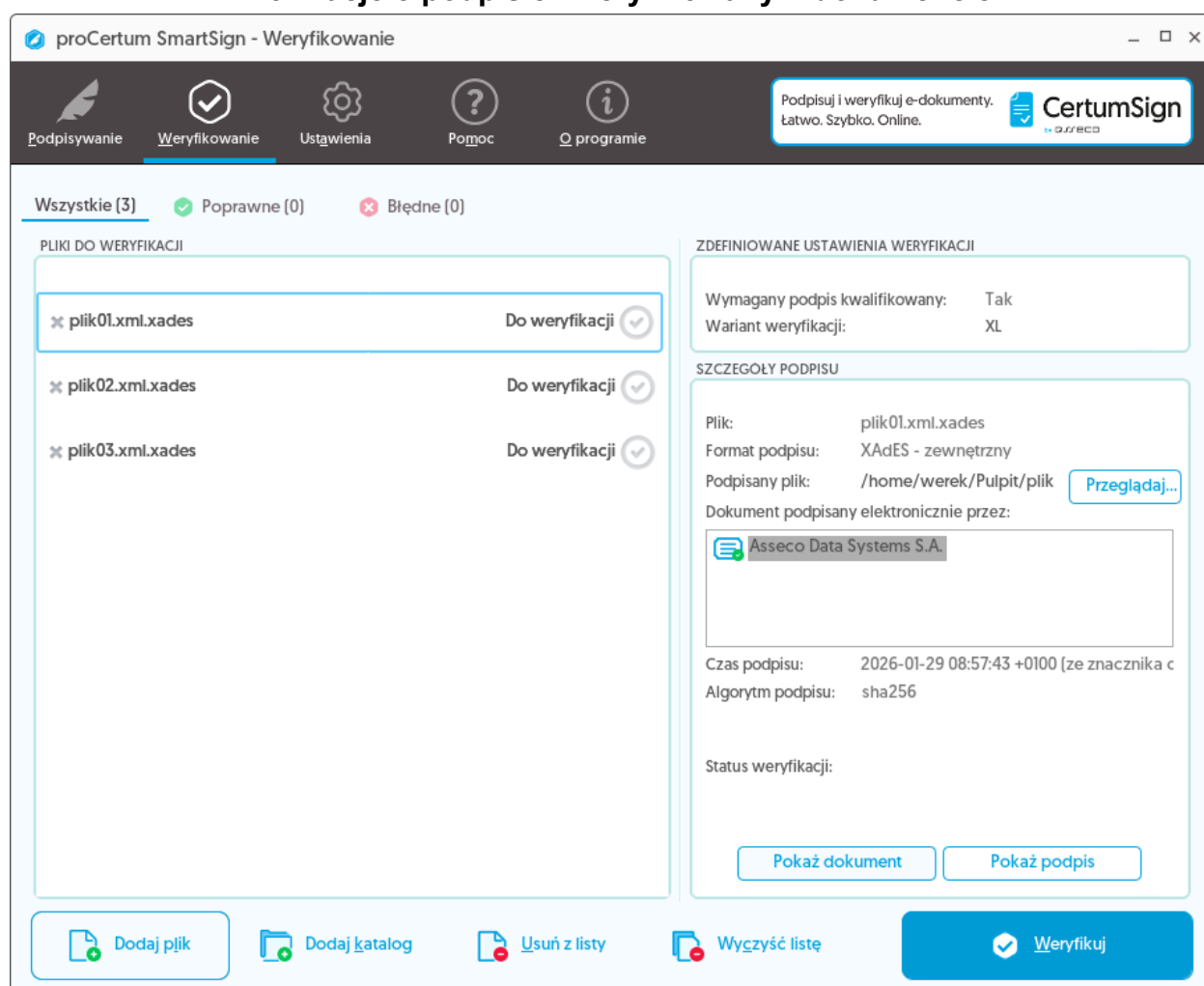
Rysunek 43: Zakładka Weryfikowanie – Lista elementów do weryfikacji
