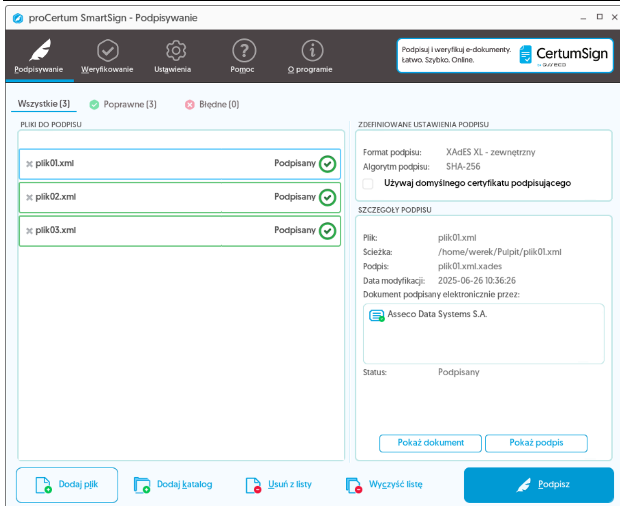
Rysunek 25: Zakładka Podpisywanie – wykonany podpis
