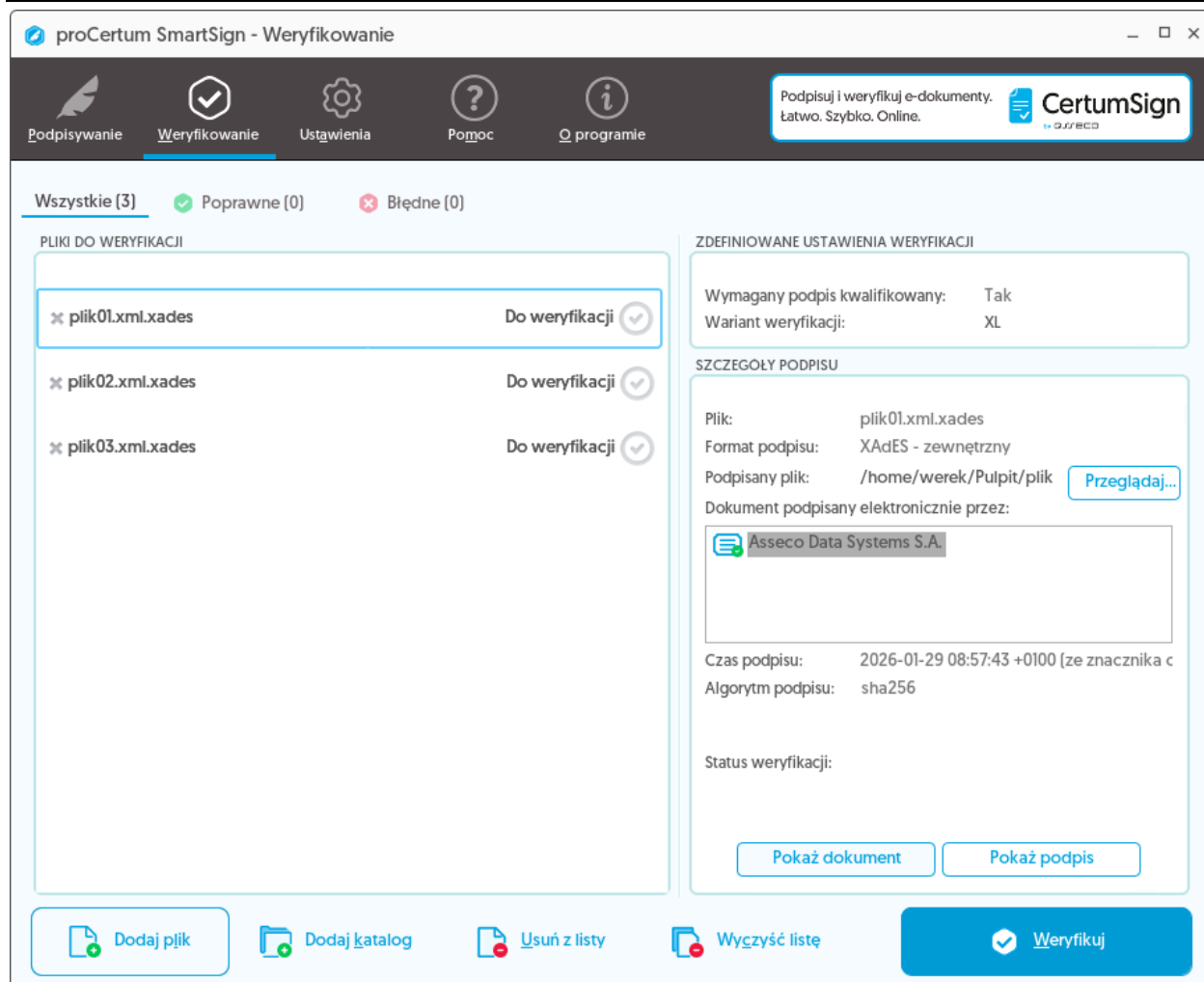
Rysunek 45: Zakładka Weryfikowanie – Lista elementów do weryfikacji
