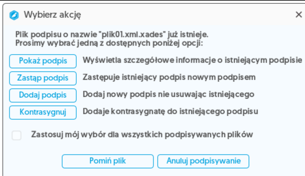
Rysunek 28: Okno wyboru akcji przy obecnym już co najmniej jednym podpisie
