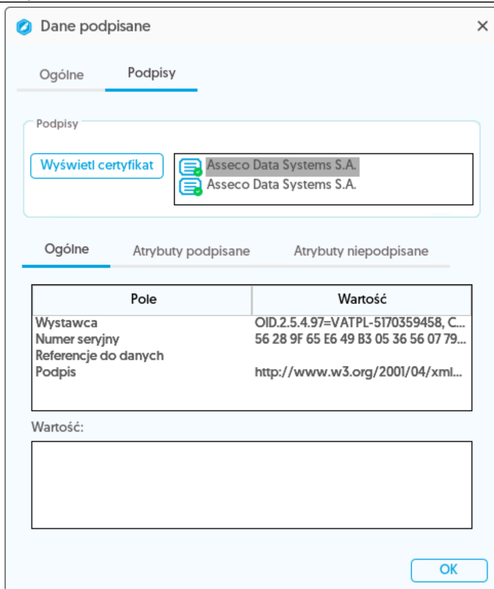
Rysunek 30: Dane podpisane - zakładka podpis dla podpisu wielokrotnego
