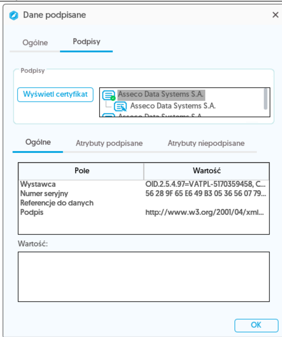
Rysunek 35 Dane podpisane - zakładka podpis dla kontrasygnaty
